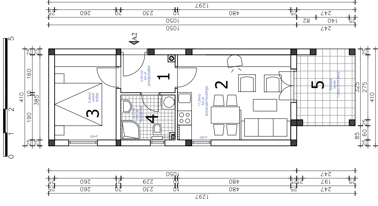
TLOCRT STANA A2 1:100
